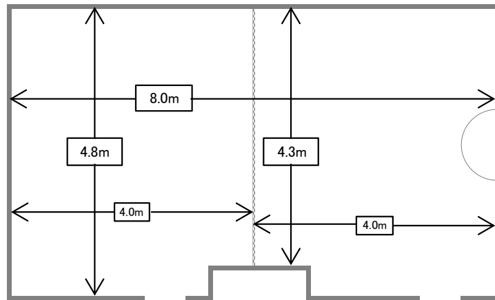
寸法図
